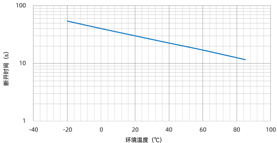
SHJ 22 A 温度-时间曲线
