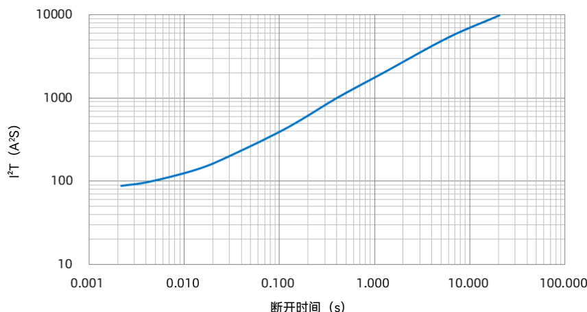
SHJ 15 A I^2t -t 曲线
