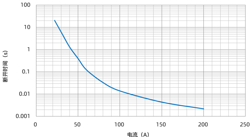
SHJ 15 A 电流-时间曲线
