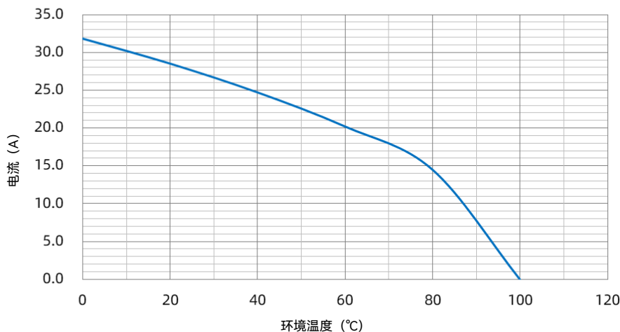
SHJ 22 A 载流能力曲线
