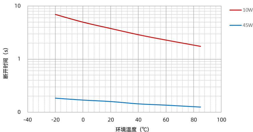
SHJ 15 A 功率-温度曲线
