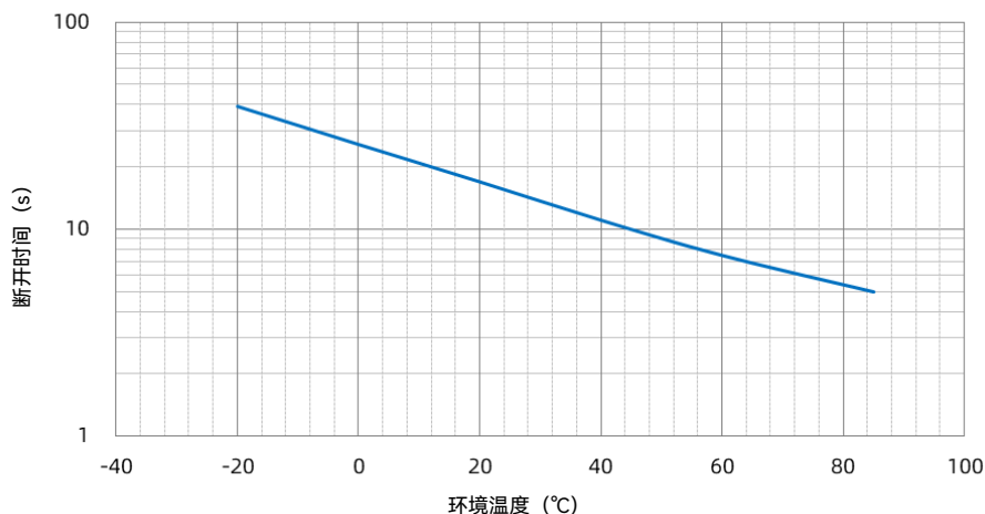
SHJ 15 A 温度-时间曲线
