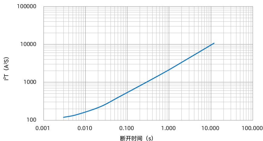
SHJ 22 A I^2t -t 曲线
