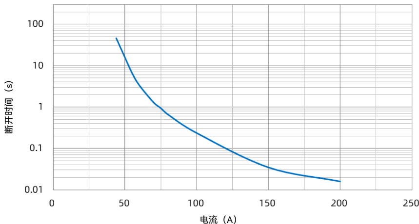
SHJ 22 A 电流-时间曲线
