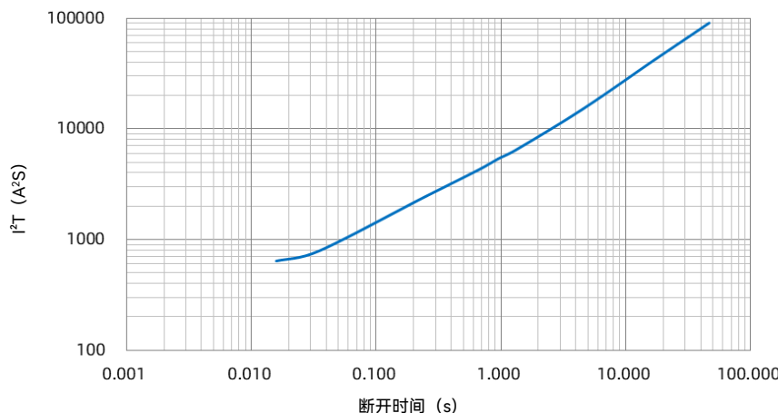
SHJ 22 A I^2t -t 曲线
