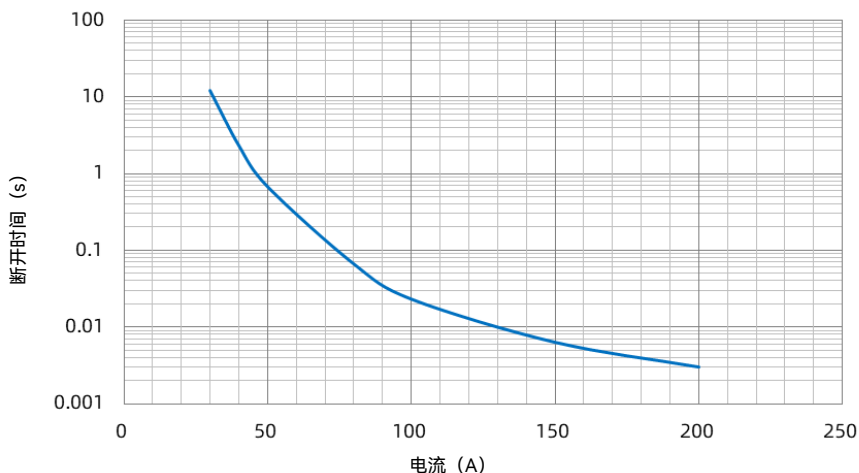
SHJ 22 A 电流-时间曲线
