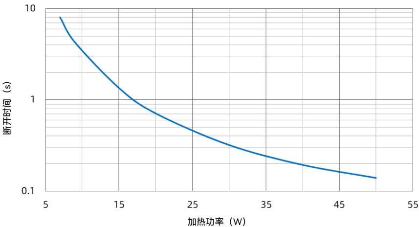
SHJ 15 A 功率-时间曲线
