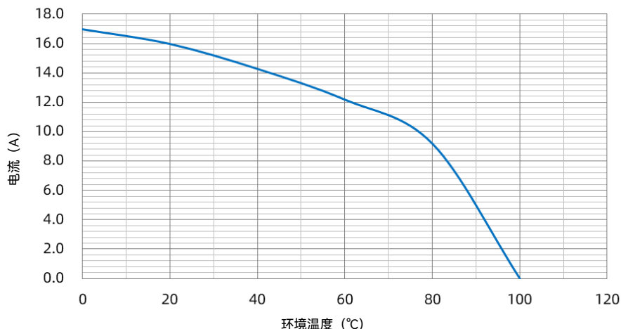
SHJ 15 A 载流能力曲线
