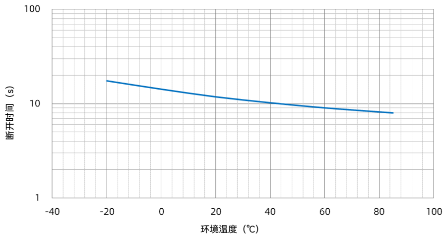
SHJ 22 A 温度-时间曲线
