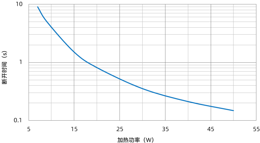
SHJ 22 A 功率-时间曲线
